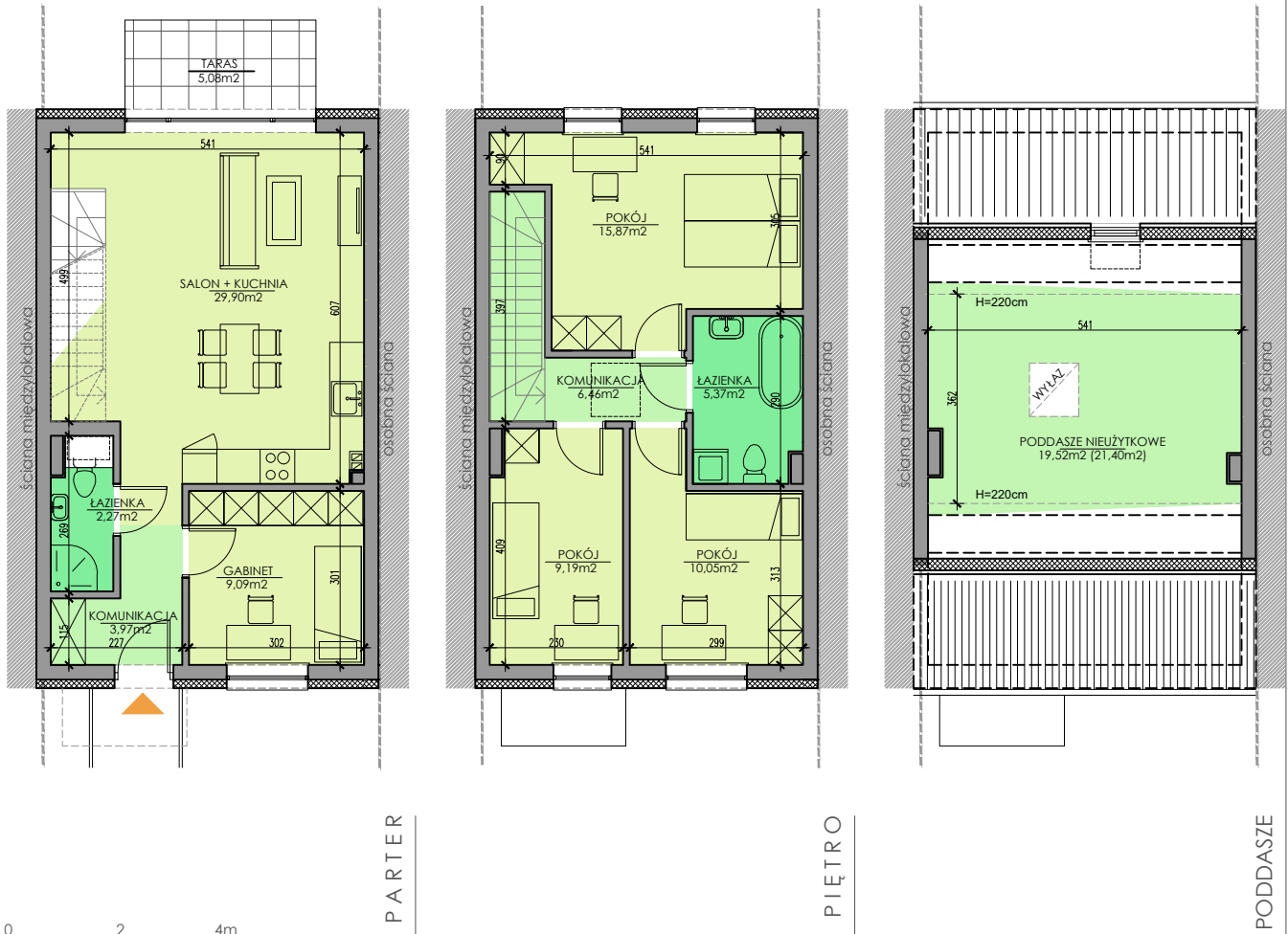
RZUTY KONDYGNACJI
